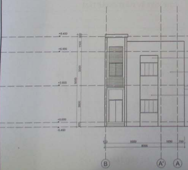
MẶT ĐÚNG TRỤC A
