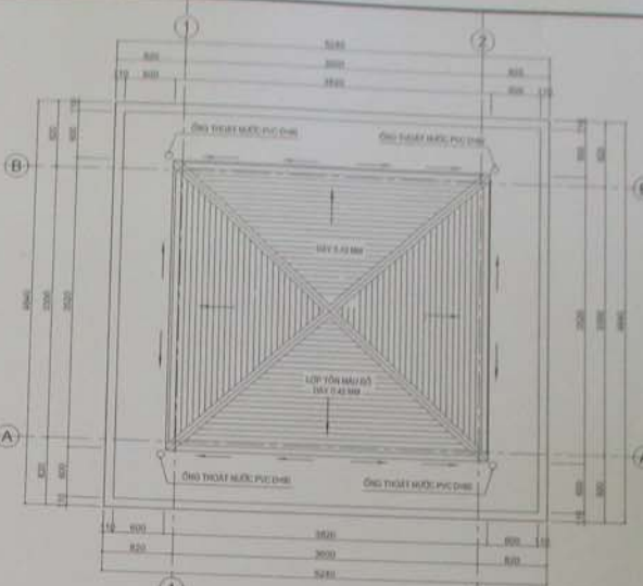
MẶT BẰNG MÁI NHÀ BẢO VỆ
