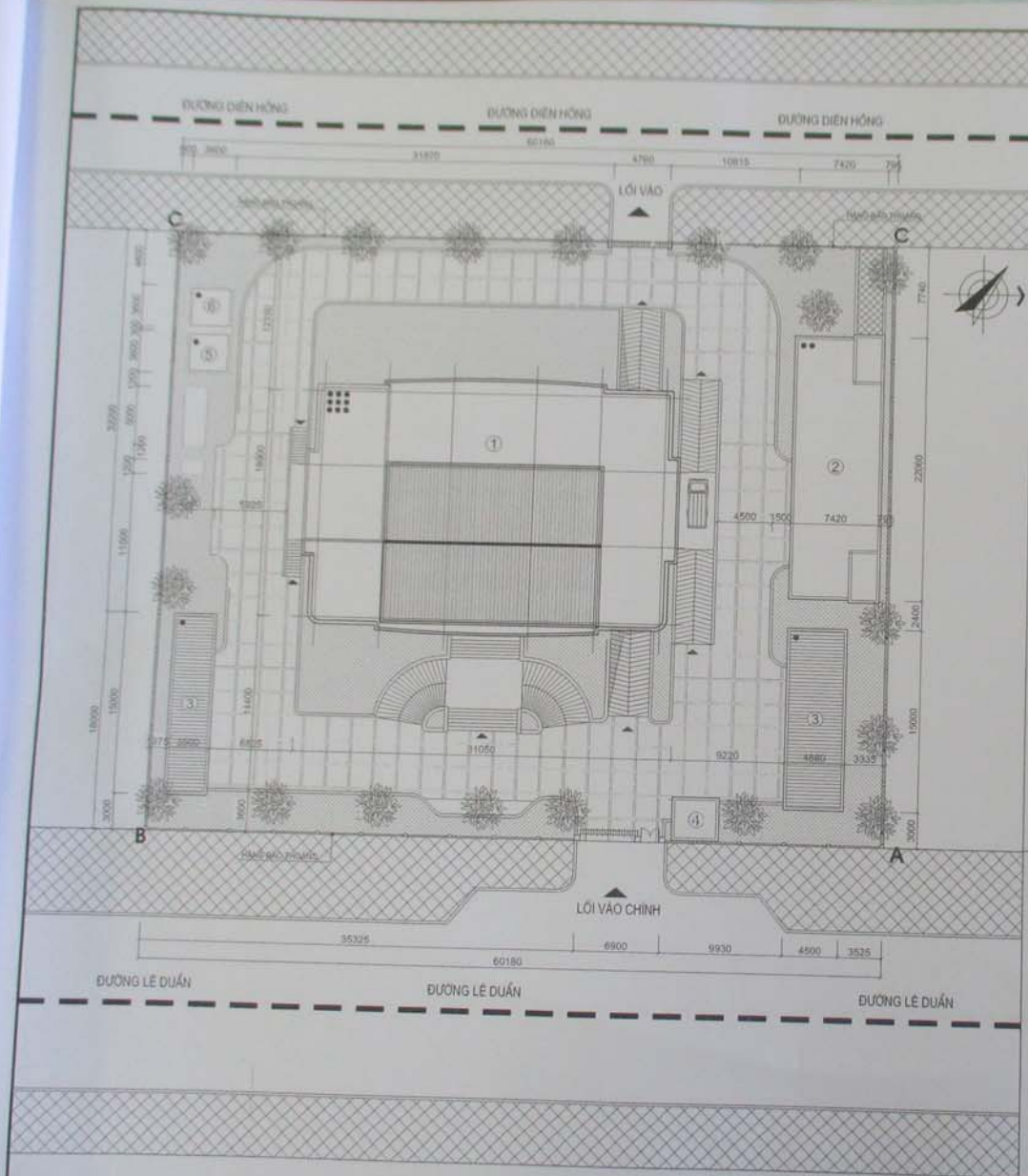
MẶT BẰNG TỔNG THỂ CÔNG TRÌNH
