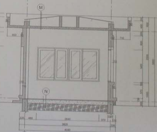
MẶT CẮT 1 - 1
