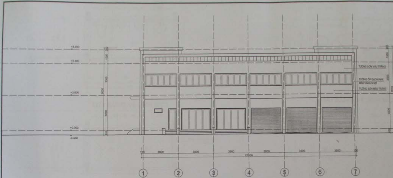
MẶT ĐÚNG TRỤC 1-7
