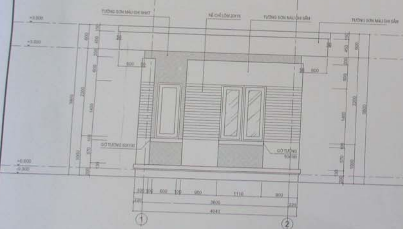
MẶT ĐỨNG TRỰC 1 - 2
